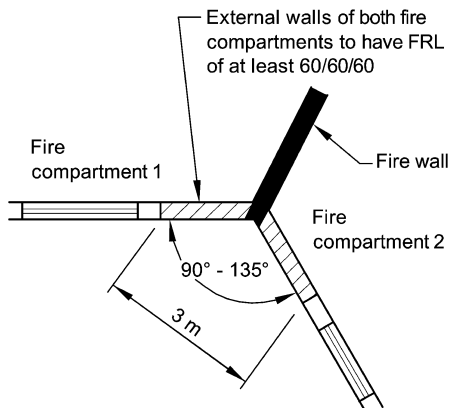
(d) External walls between 90° - 135°
