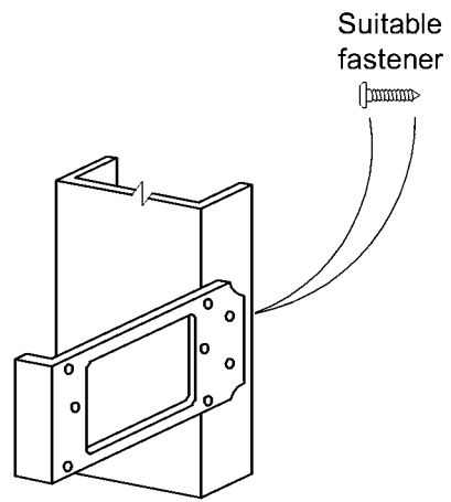
(d) Switch and power point backing plate
