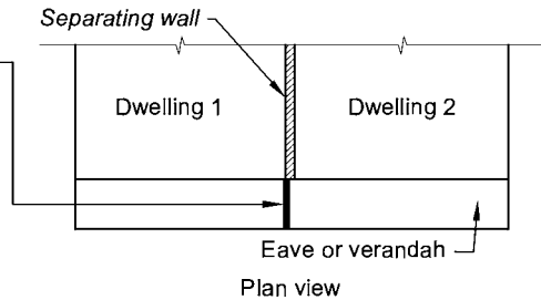
(d) Separation of eave / verandah
