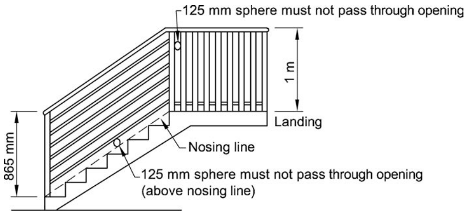
(a) Stairways - D2-16(d)
