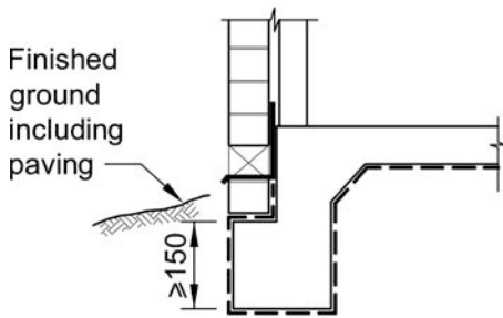
(b) Deep edge rebate alternative
