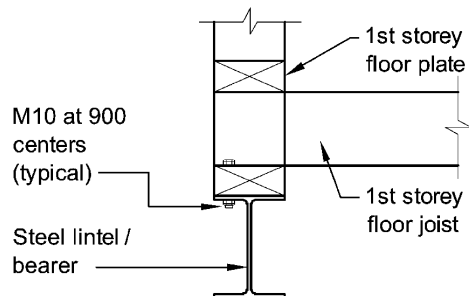
(d) Floor - example B
